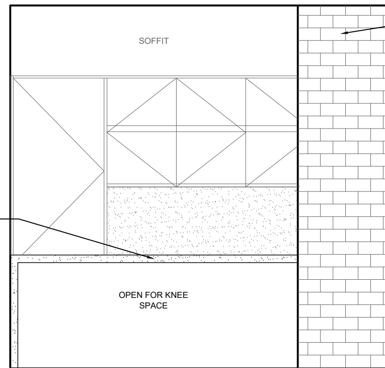
104 BAR - ELEVATION D
