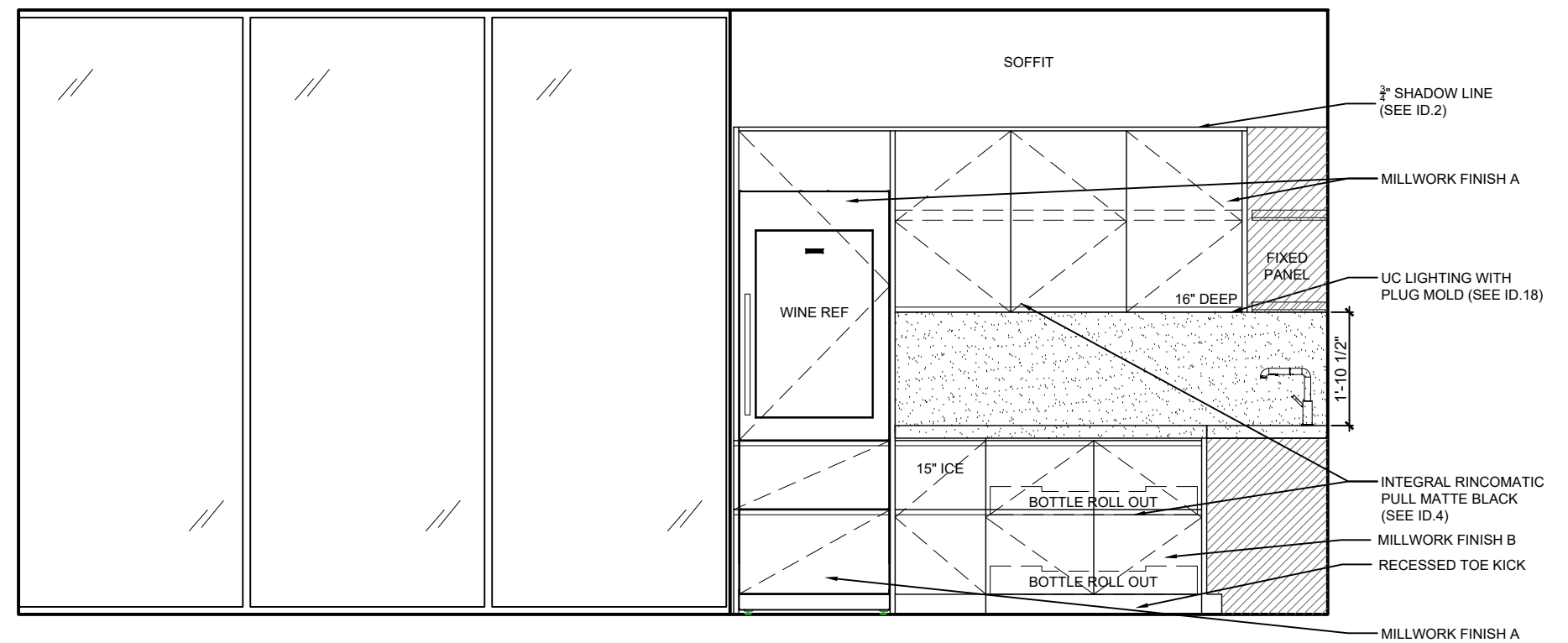
104 BAR - ELEVATION B
