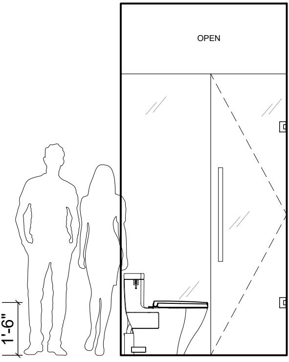
118 CASITA BATH - ELEVATION B
