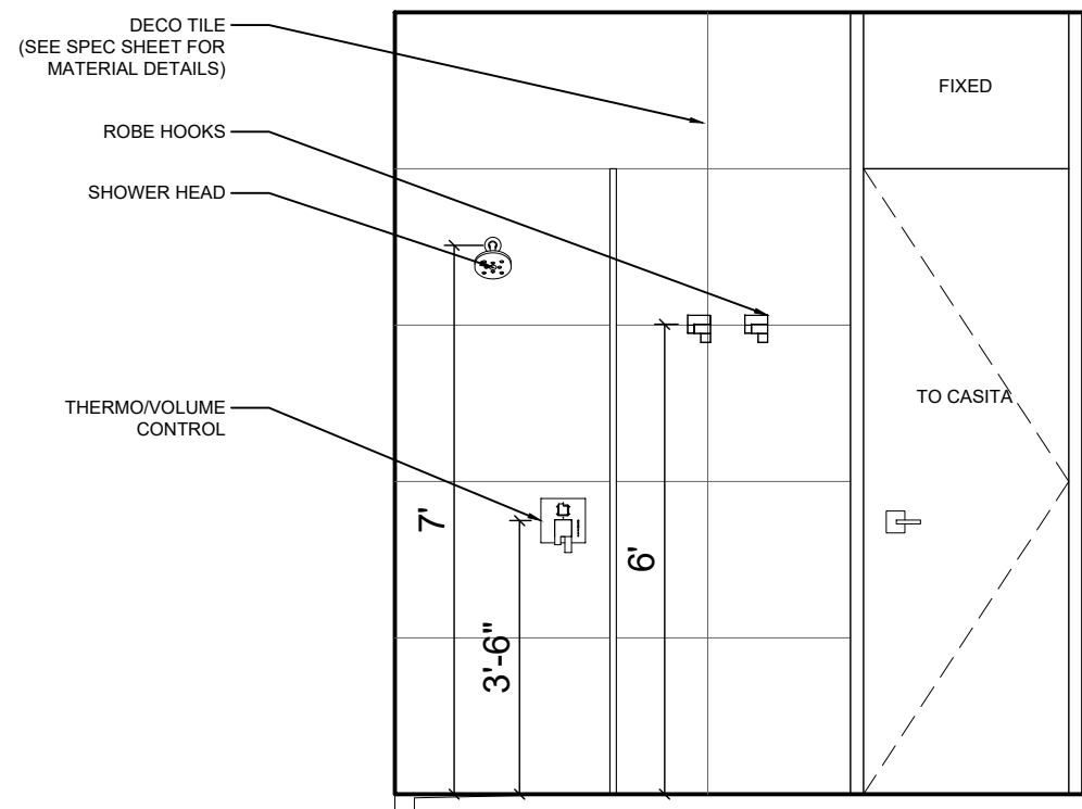
118 CASITA BATH - ELEVATION C
