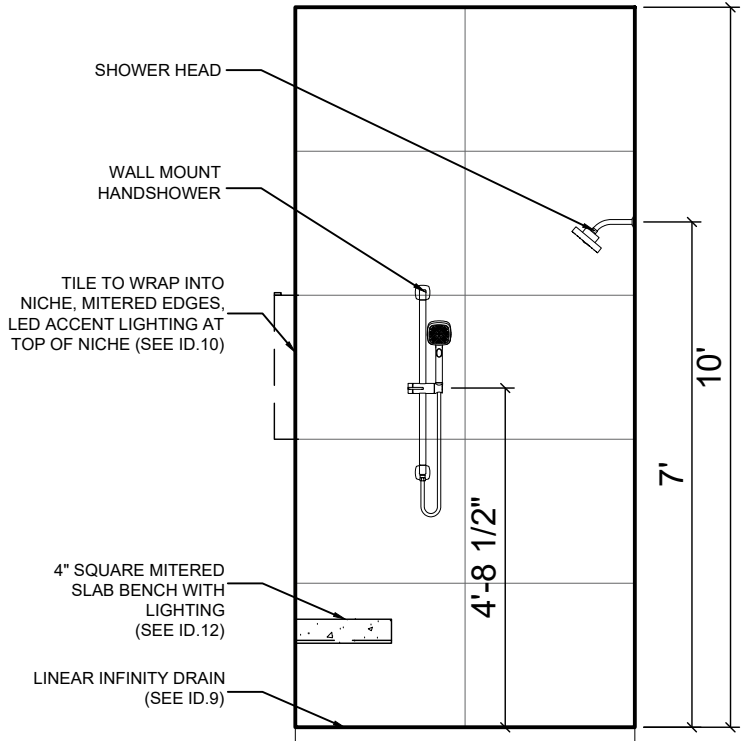
118 CASITA BATH - ELEVATION B.1
