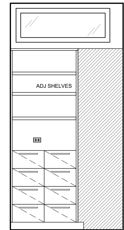
113 W.I.C 2 - ELEVATION D
