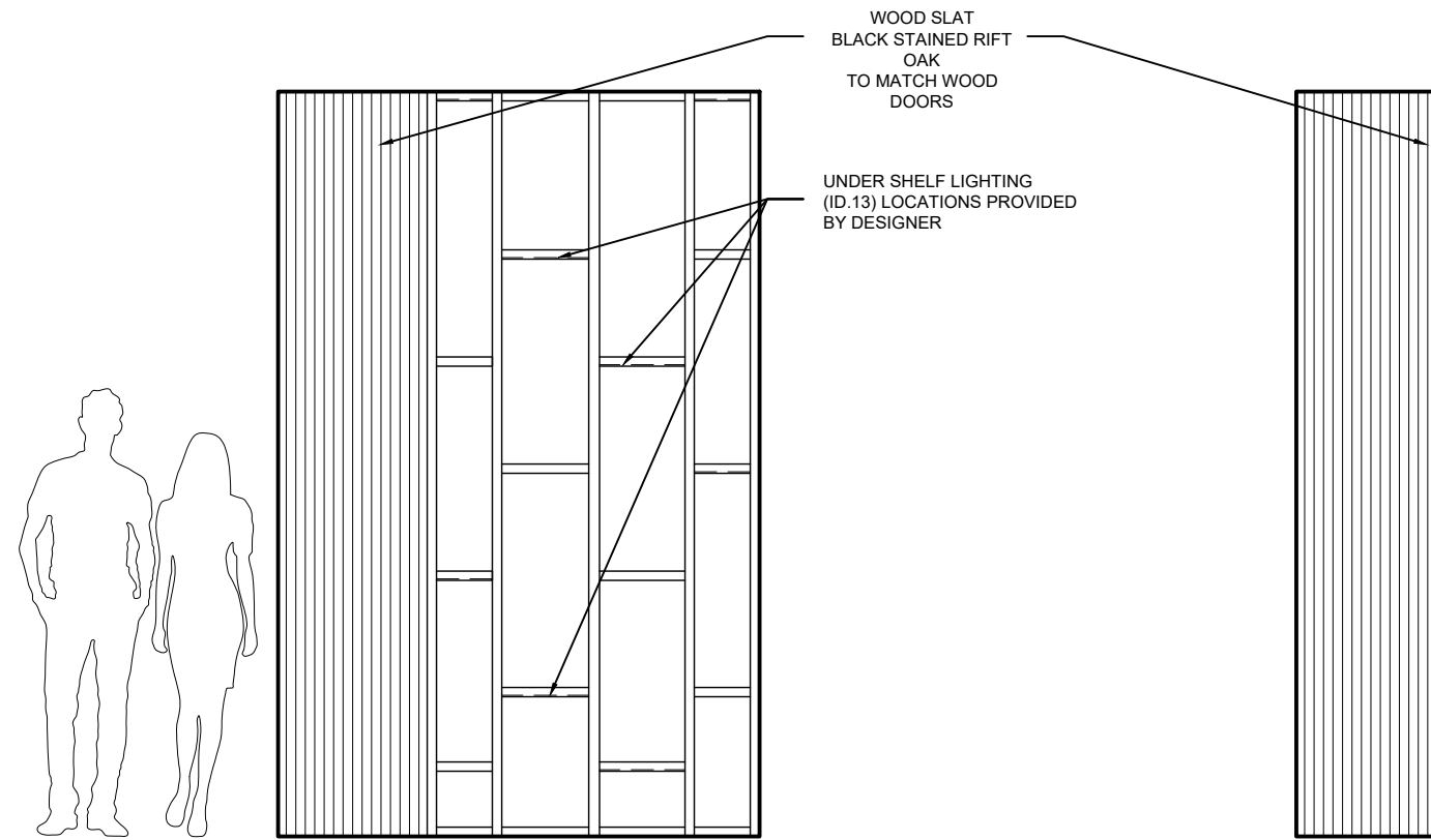
204 VIEWING LOFT - ELEVATION E
